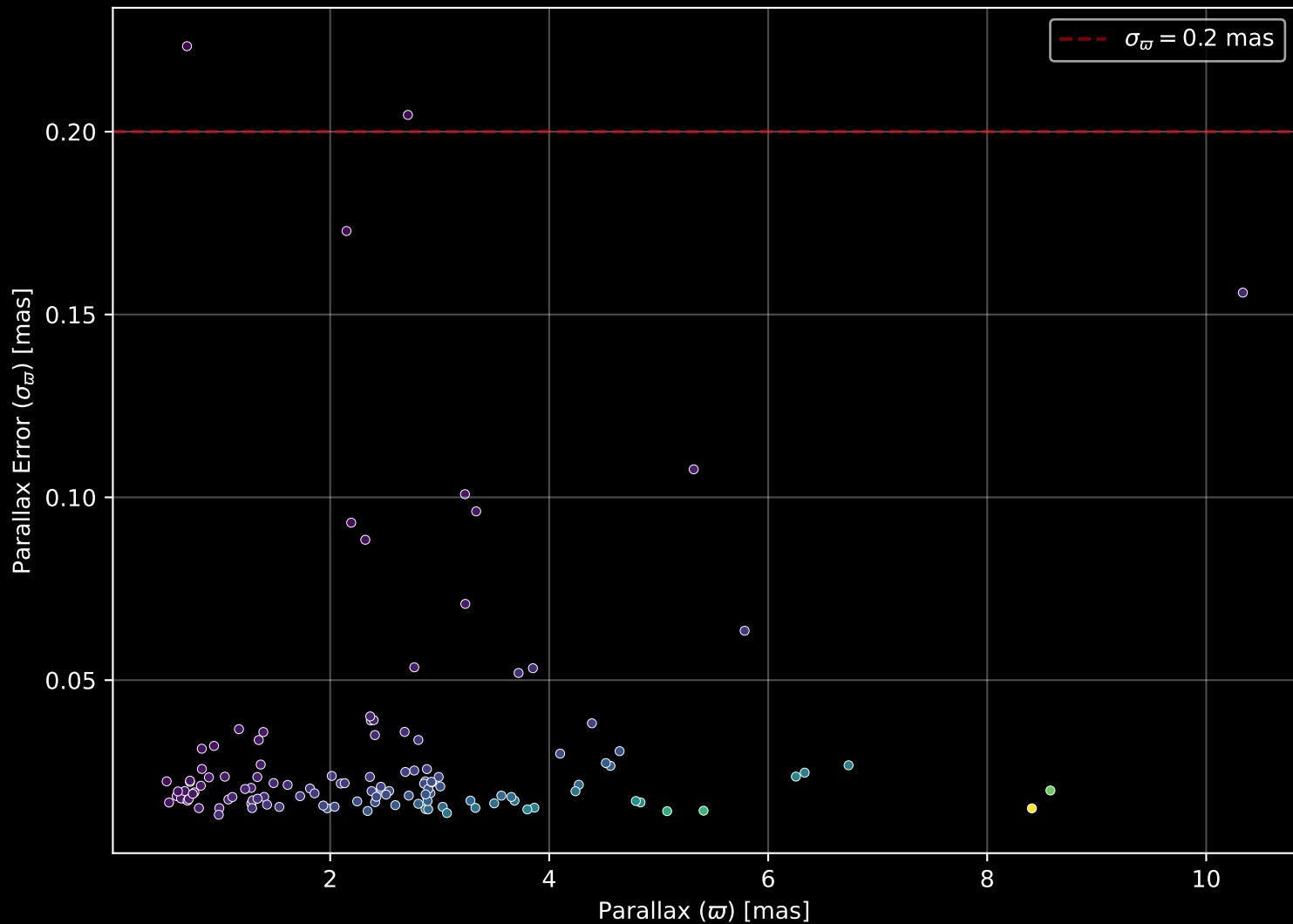
GALAH DR4 Field: [2878] Parallax Quality (n= 124)
