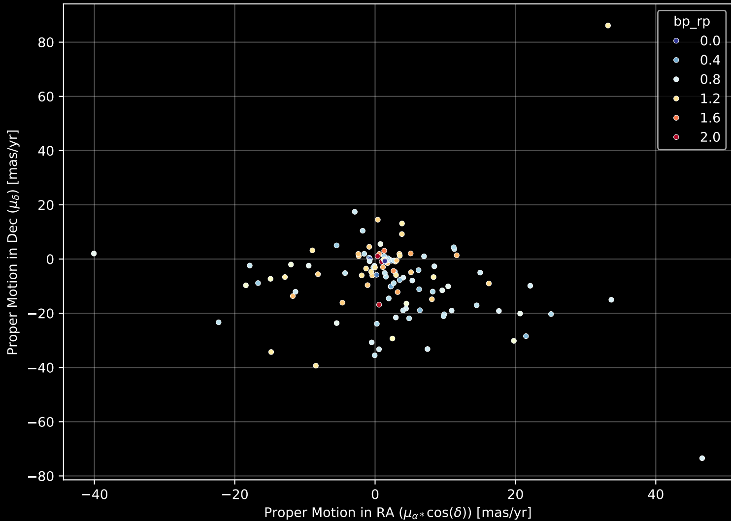
GALAH DR4 Field: [2878] Proper Motion Diagram (n= 124)
