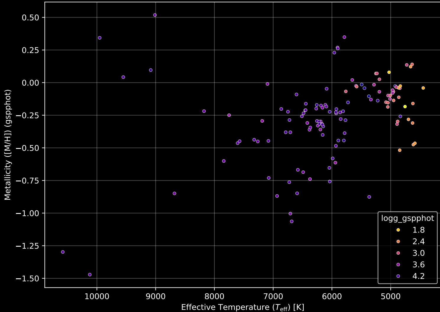
GALAH DR4 Field: [2878] Stellar Population Parameters (n= 124)
