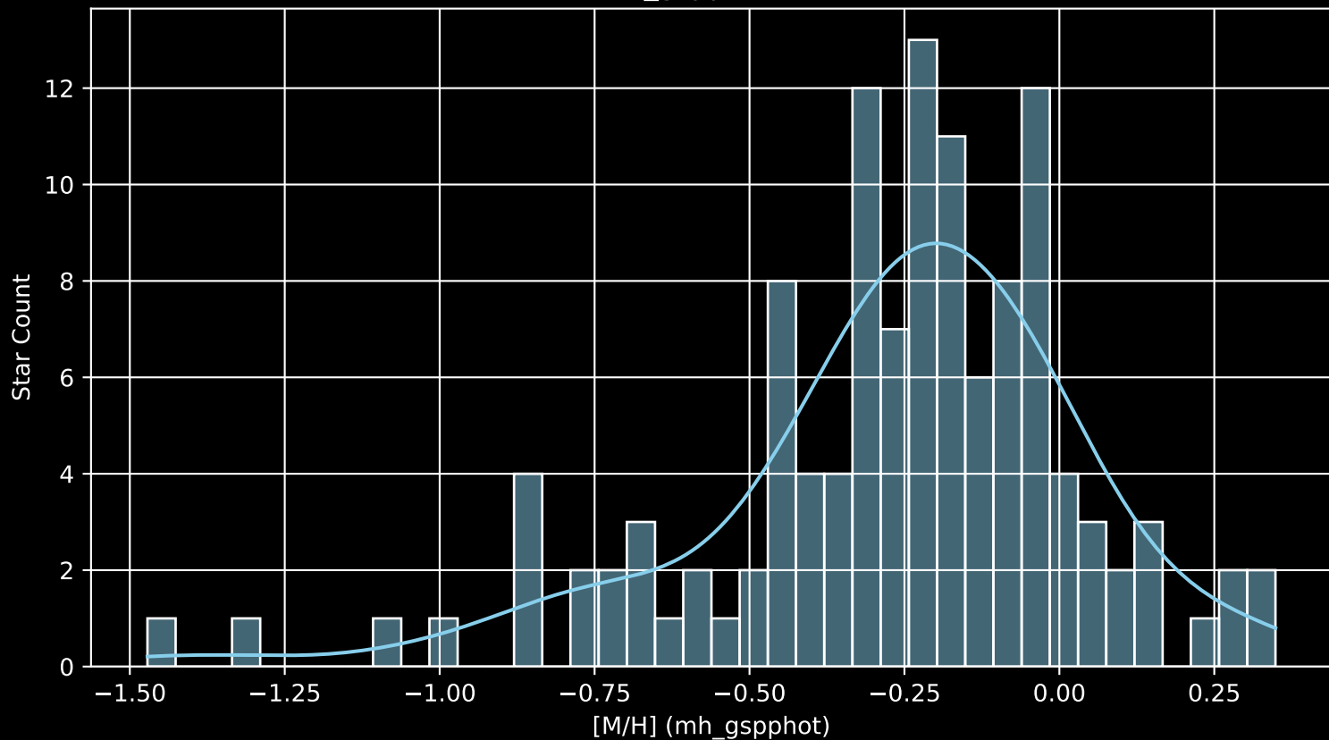
GALAH DR4 Field: [2878] [M/H] (mh_gspphot) (n= 123)
